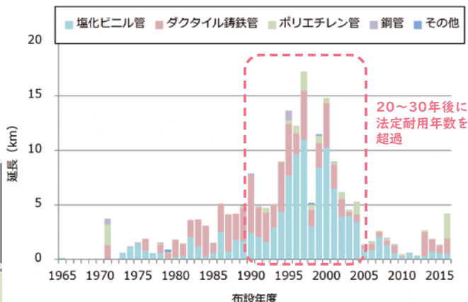
管種及び布設年度ごとの管路延長
