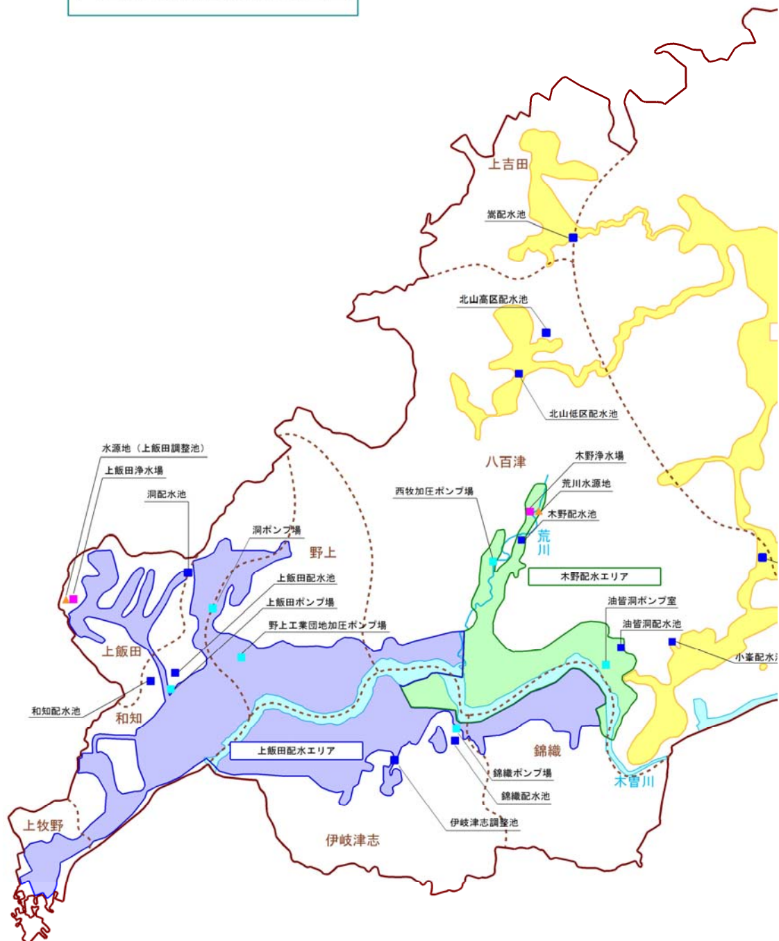
八百津町水道施設位置図
