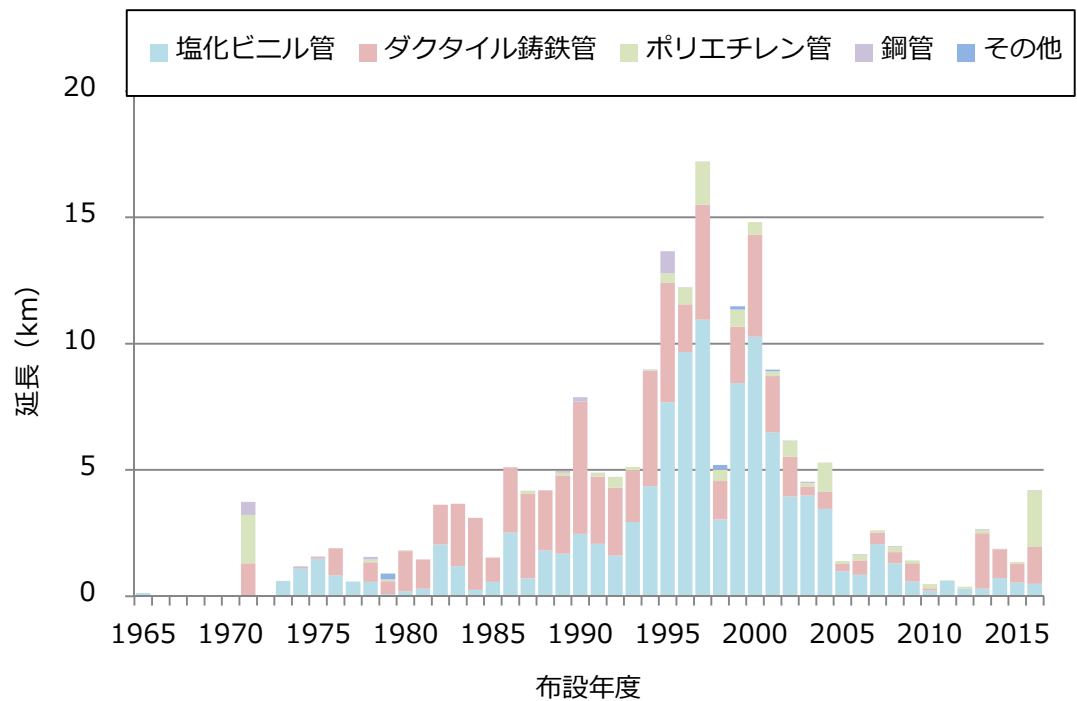
図 管種及び布設年度ごとの管路延長
