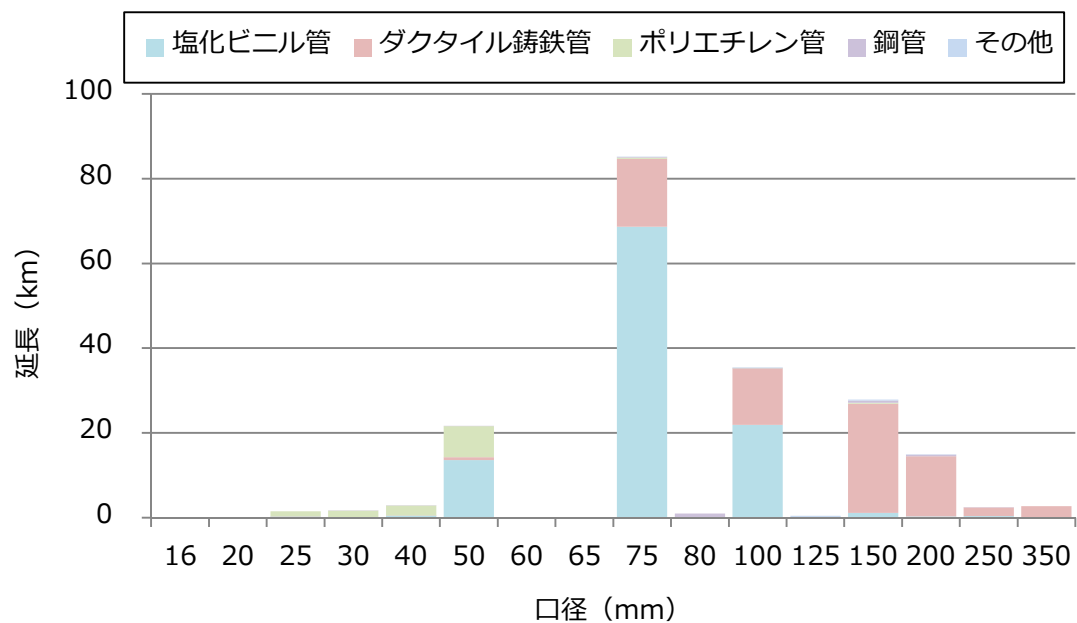
図 管種及び口径ごとの管路延長
